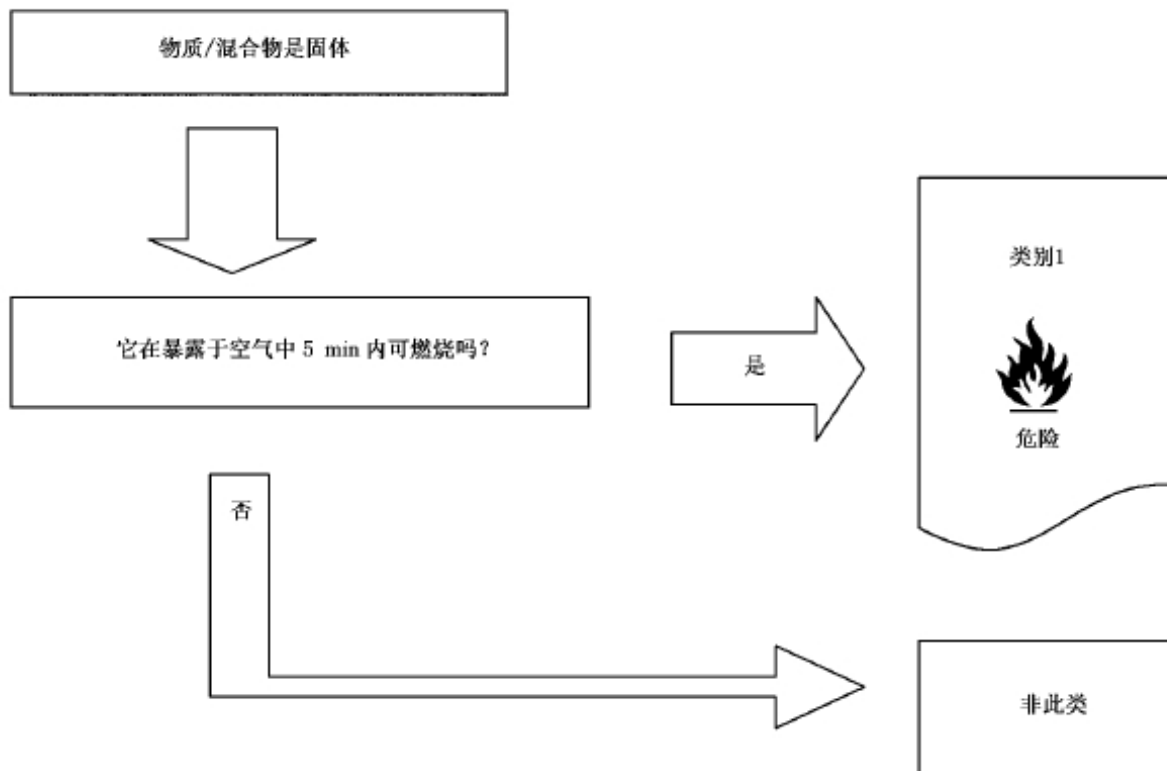
图 A.1 自燃固体判定逻辑
