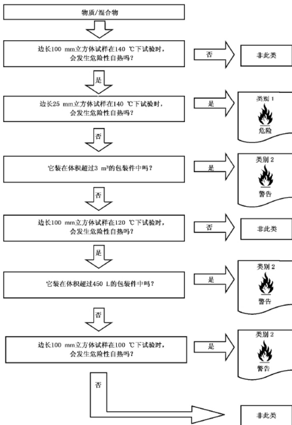
图 A.1 自热物质和混合物判定逻辑
