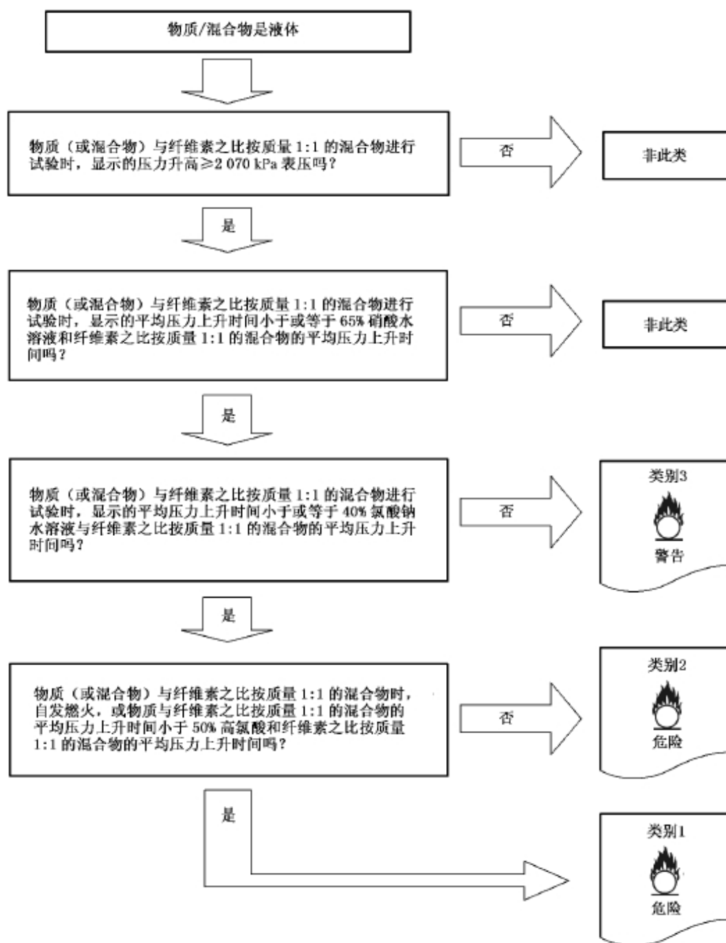
图 A.1 氧化性液体判定逻辑
