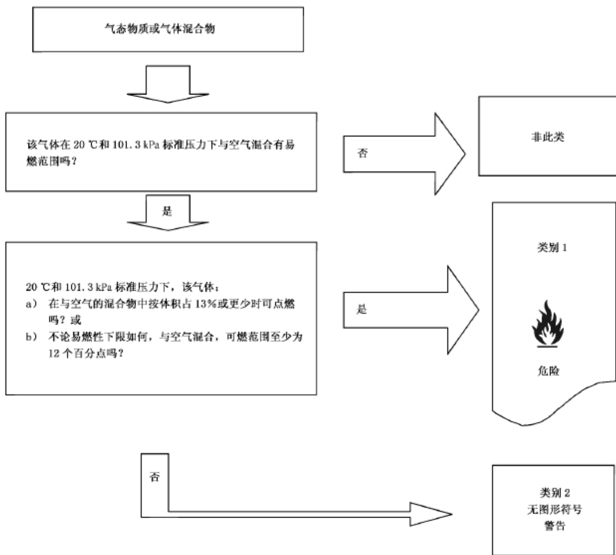
图 A.1 易燃气体的判定逻辑
