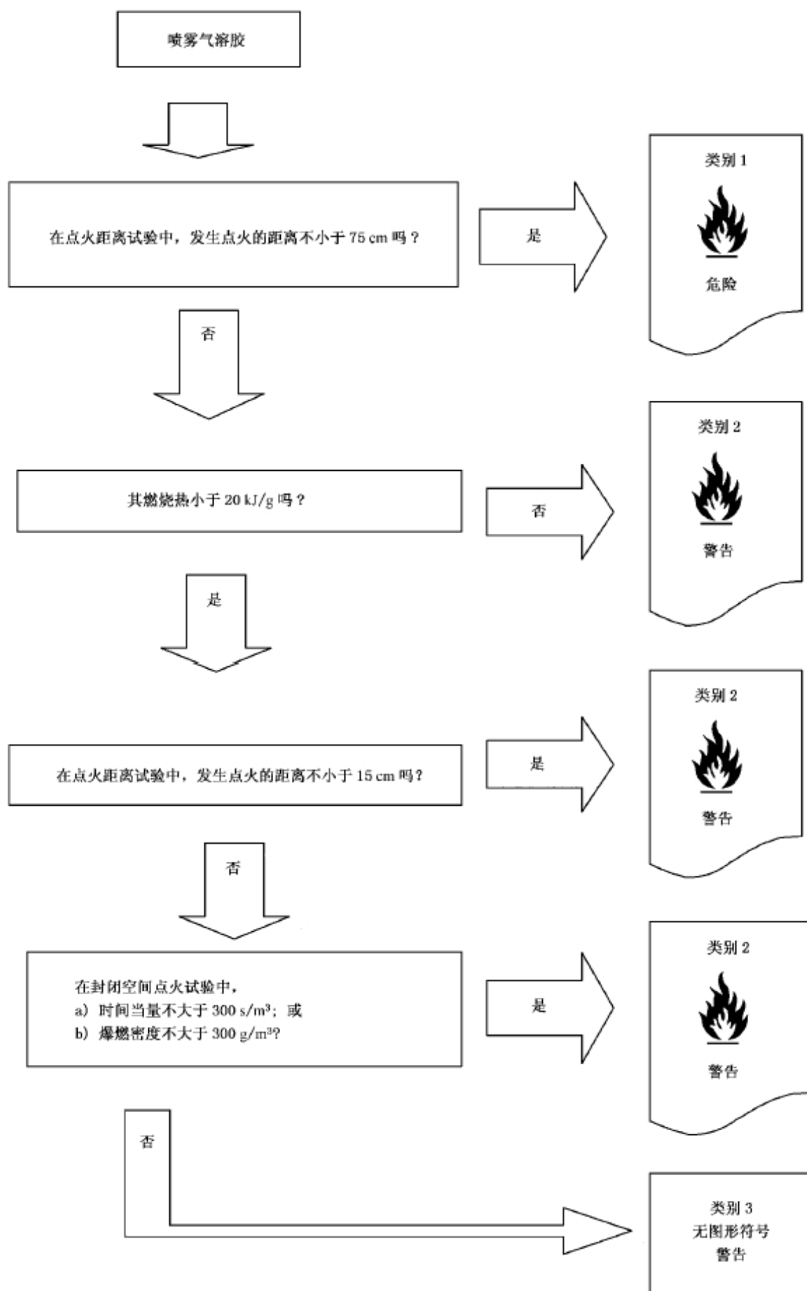
图 A.2 喷雾气溶胶判定逻辑
