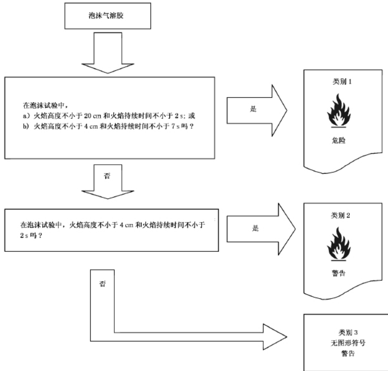
图 A. 3 泡沫气溶胶判定逻辑
