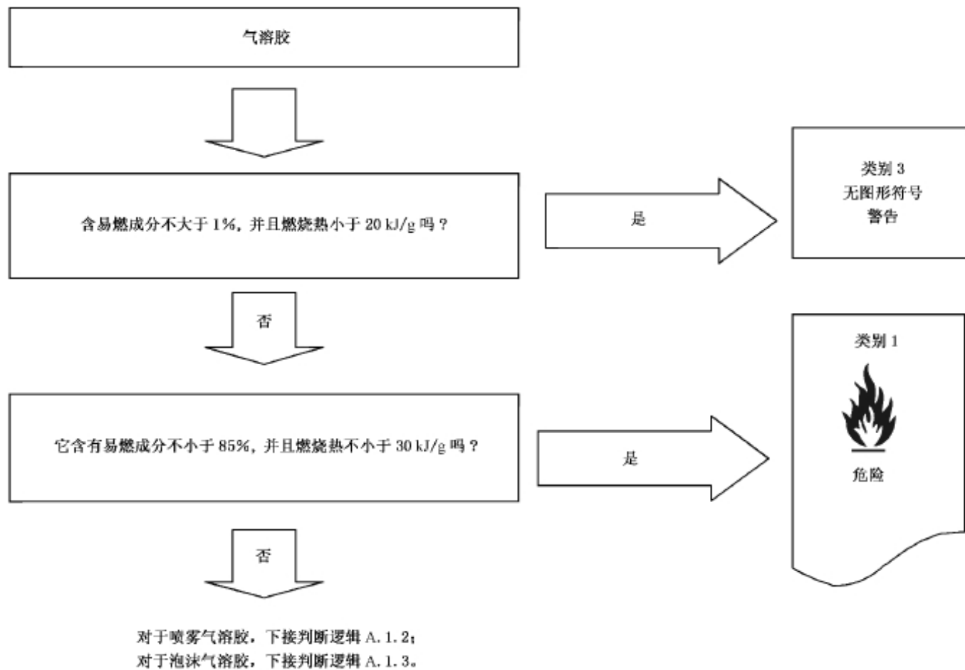
图 A.1 气溶胶的判定逻辑
