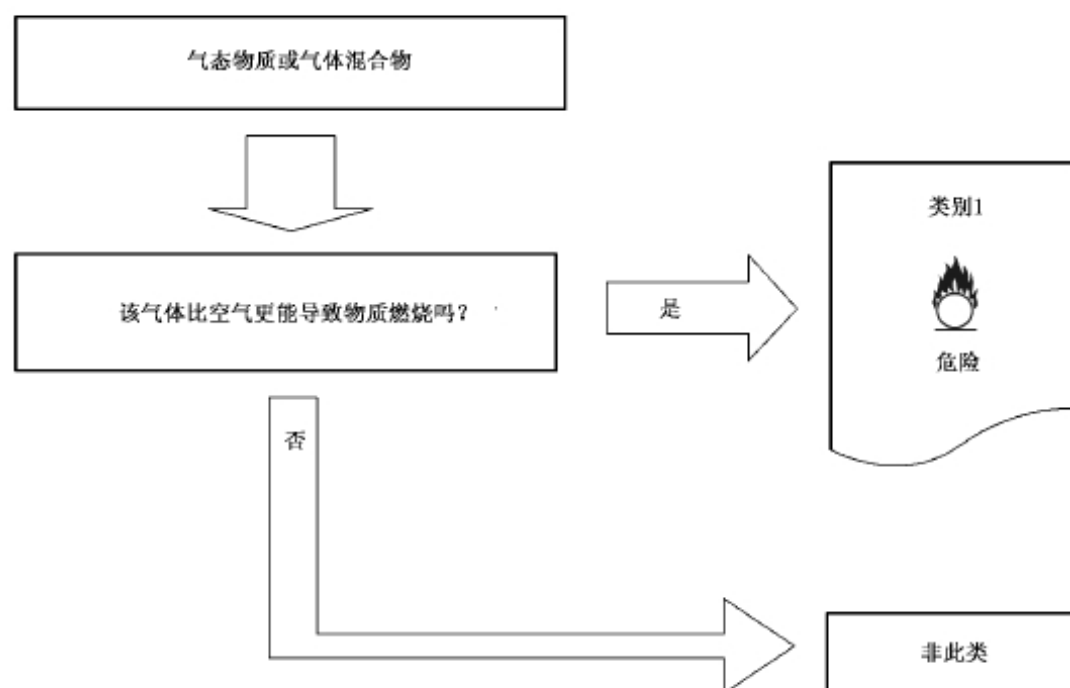
图 A.1 氧化性气体判定逻辑
